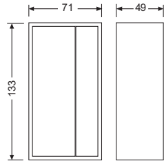
尺寸 (mm)
