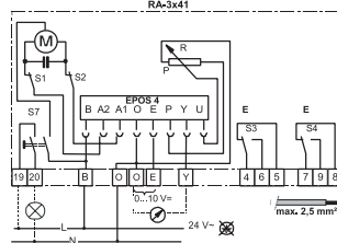
比例控制型接线图
